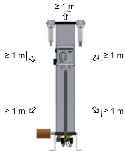
Distance nécessaire vers le haut et sur les côtés = min. 1 m
